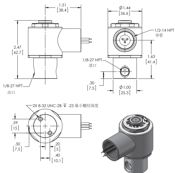
EL50 系列 EL52 二位二通常闭型 防爆型
